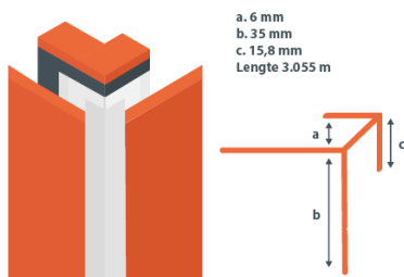
TYPE E Buitenhoekprofiel
